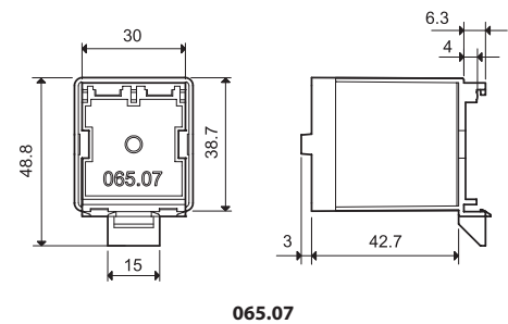
Адаптер 35 мм рейки (EN 60715) для реле типов 65.31.xxxx.xxx9
