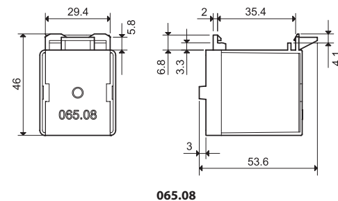
Адаптер 35 мм рейки (EN 60715) для реле типов 65.31.xxxx.xxx9
