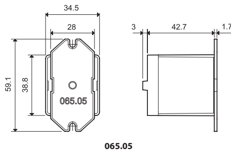
фланцевый адаптер крепления для реле типов 65.31.xxxx.xxx9
